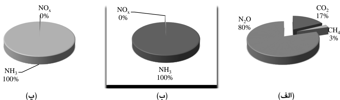
شکل ۲- سهم انتشار آلاینده‌ها برای گروه‌های تأثیر الف) گرمایش جهانی، ب) اسیدیته و پ) اوتریفیکاسیون خشکی به ازای یک واحد عملکردی نظام تولید چای در گیلان
