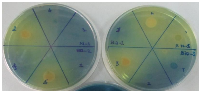
شکل ۸- پیدایش رنگ زرد یا نارنجی در جدایه‌های باکتریایی مولد سایدروفور در محیط CAS-agar (ساریخانی و انصاری ۲۰۱۵)
